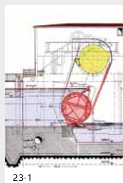
Abb. 23-1 Walzenwehr mit Aufsatzklappe
